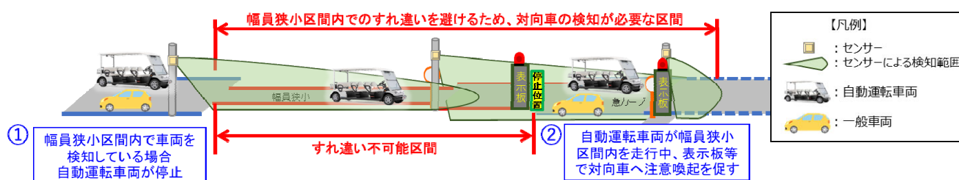
図 3 路車協調システムで支援する道路状況（幅員狭小区間でのすれ違い回避）
