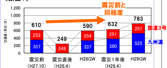
＜断面1＞
