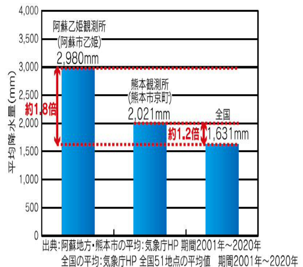
図-2 年間降雨量の比較
